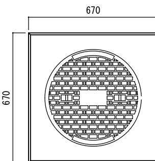
鑄鉄埋込スラブ
