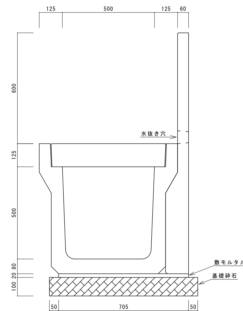
U h 礼3種500A-6 S=1/10
