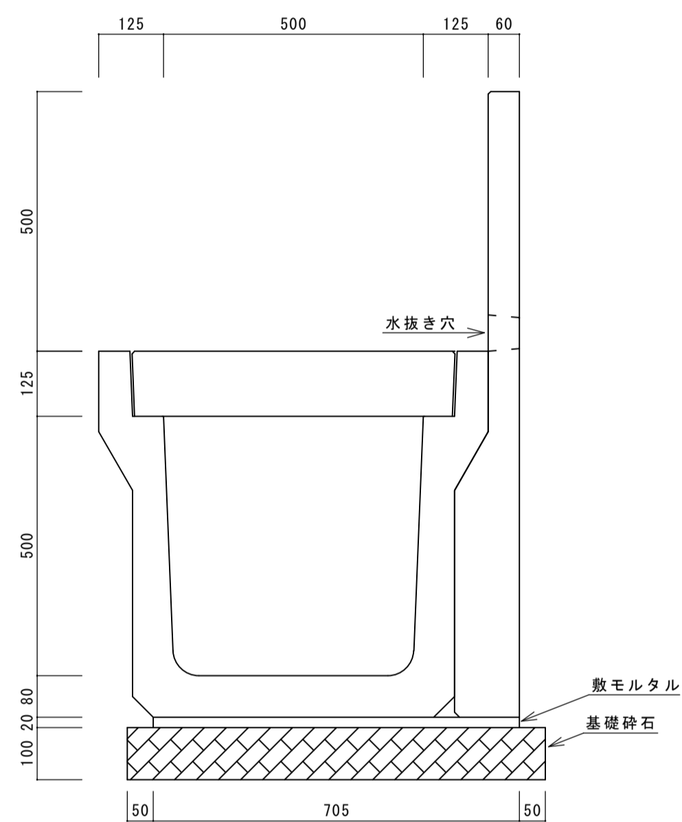
U h 礼3種500A-5 S=1/10
