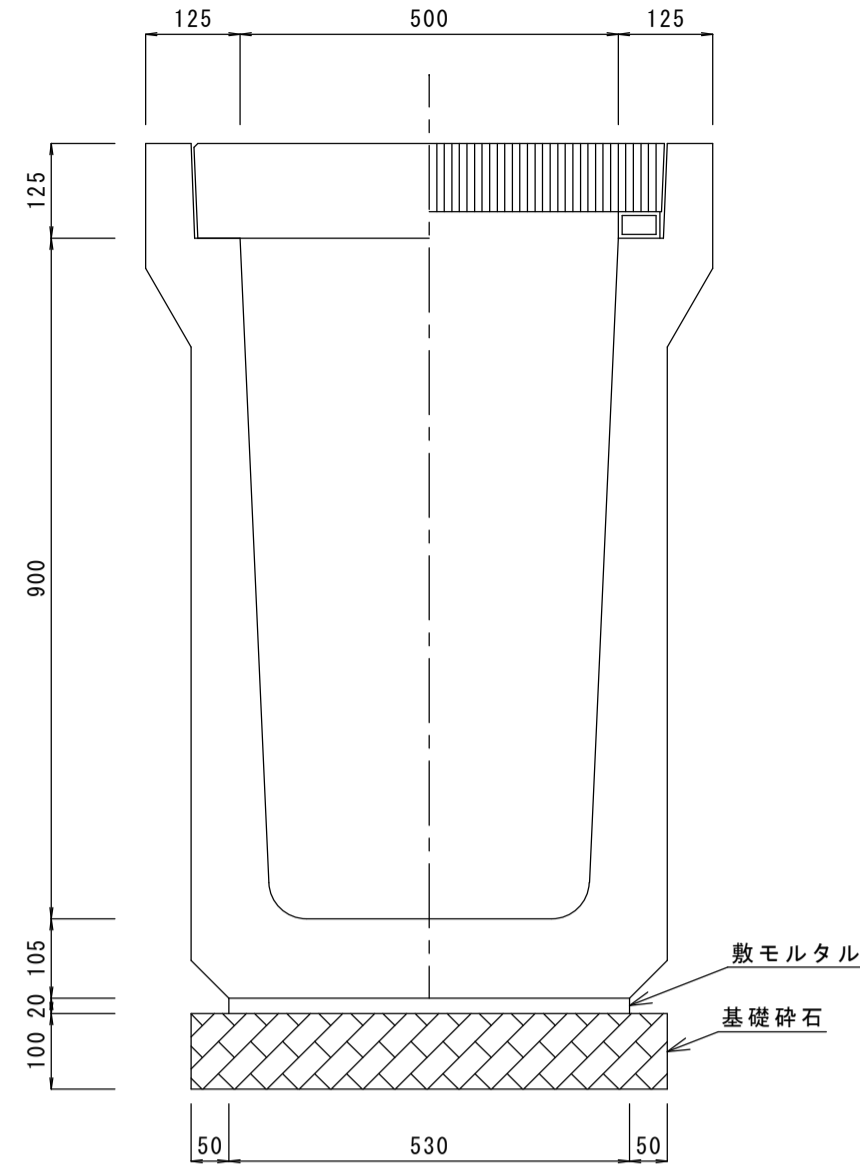
PU500*900
