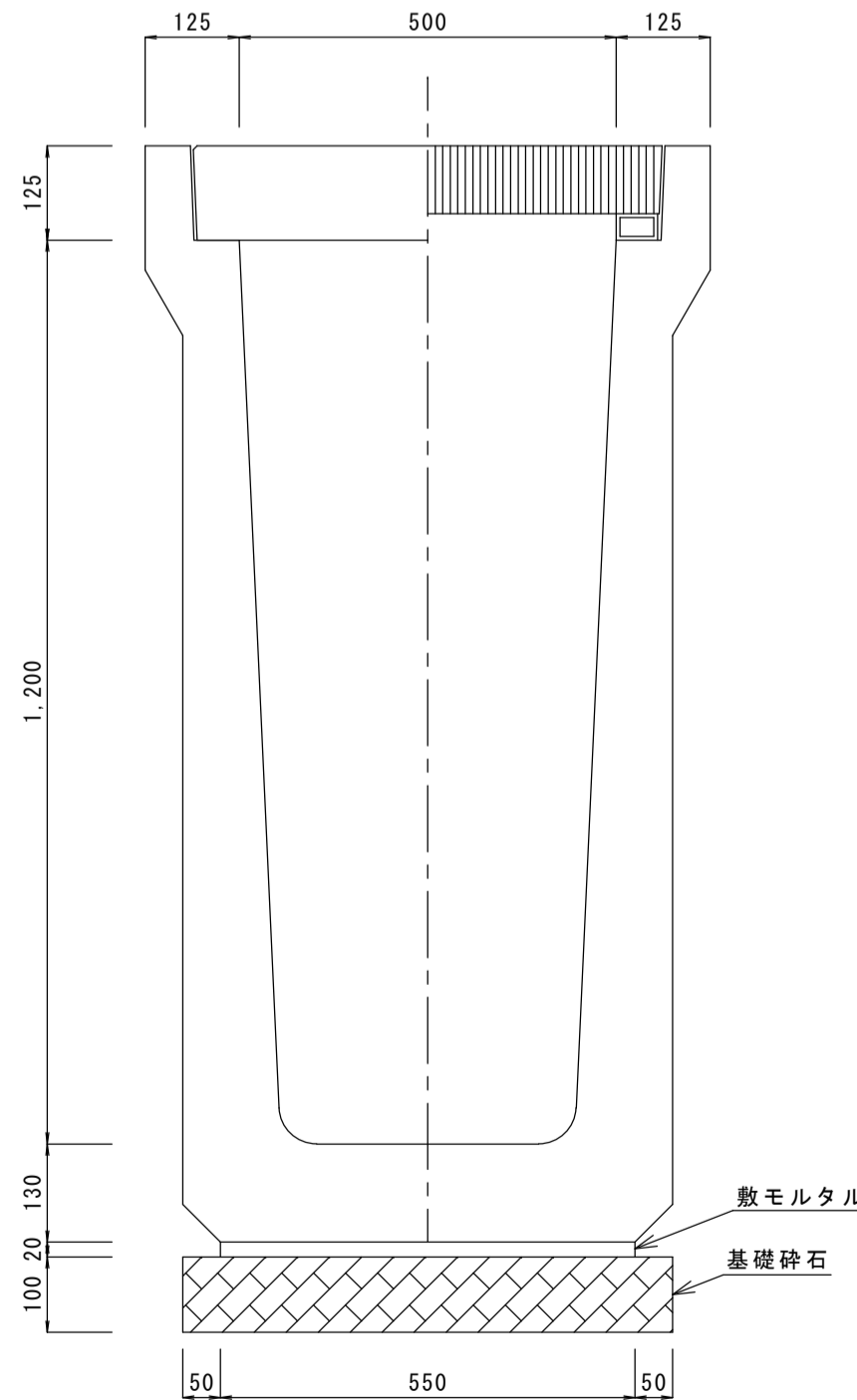
PU500*1200
