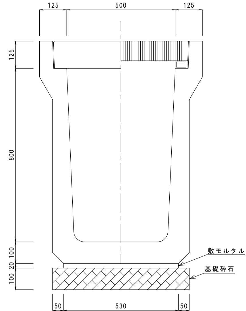
PU500*800
