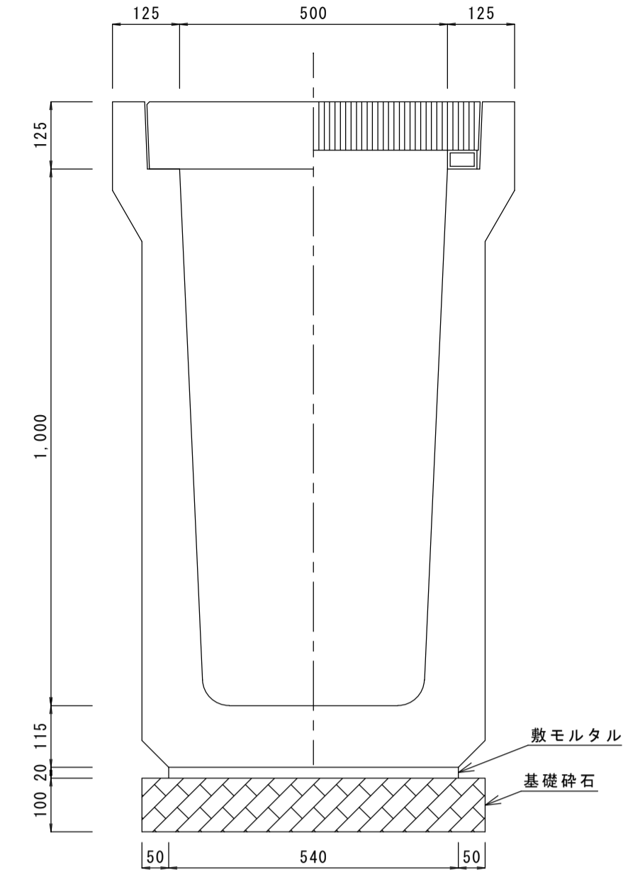
PU500*1000
