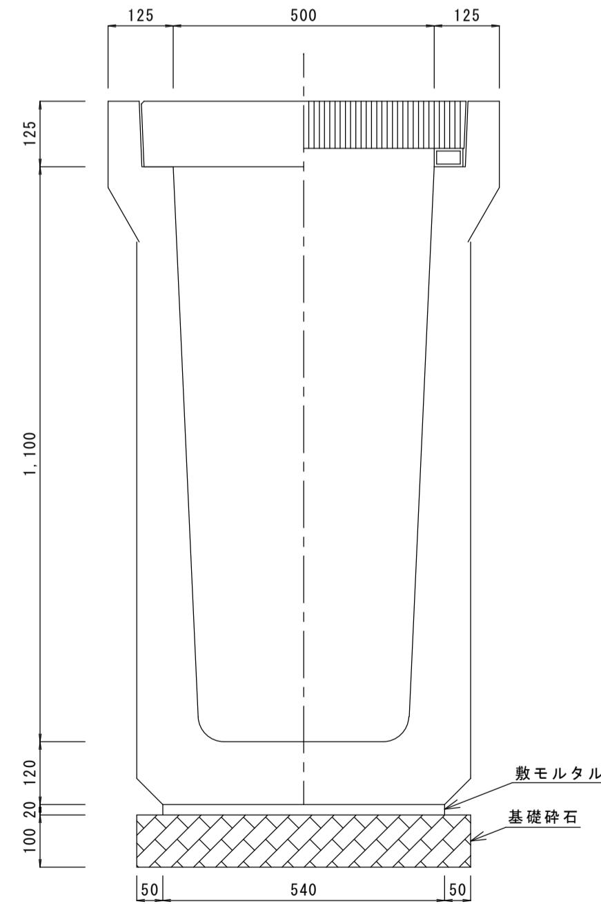
PU500*1100
