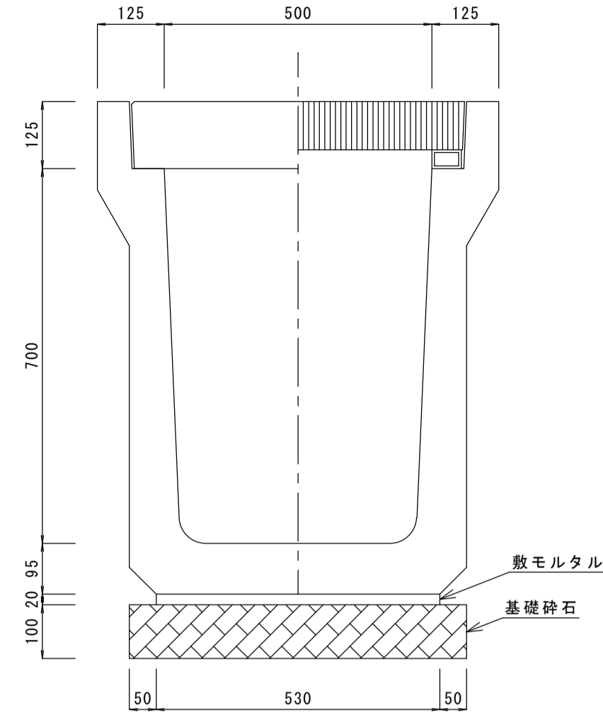
PU500*700
