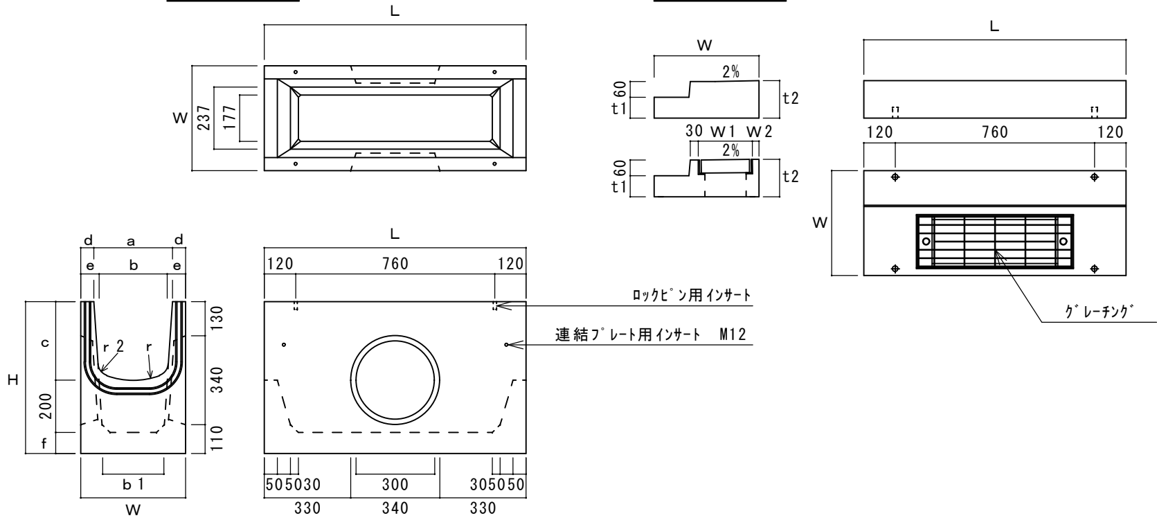
柵本体
