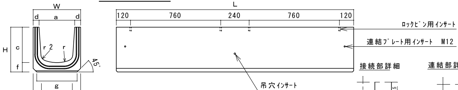
本体 側面図
