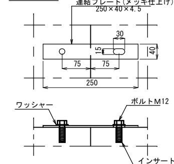
連結部詳細
