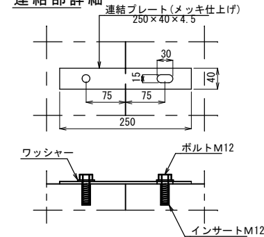
連結部詳細
