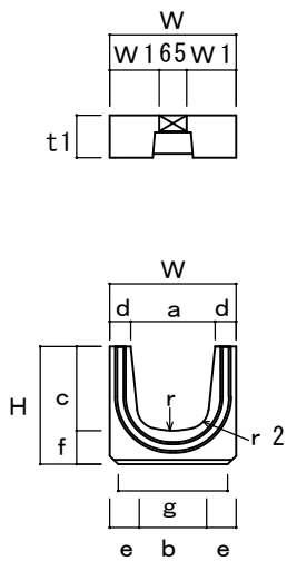
本体 側面図
