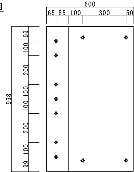
端部、調整用 平面図
