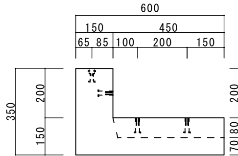
端面図
